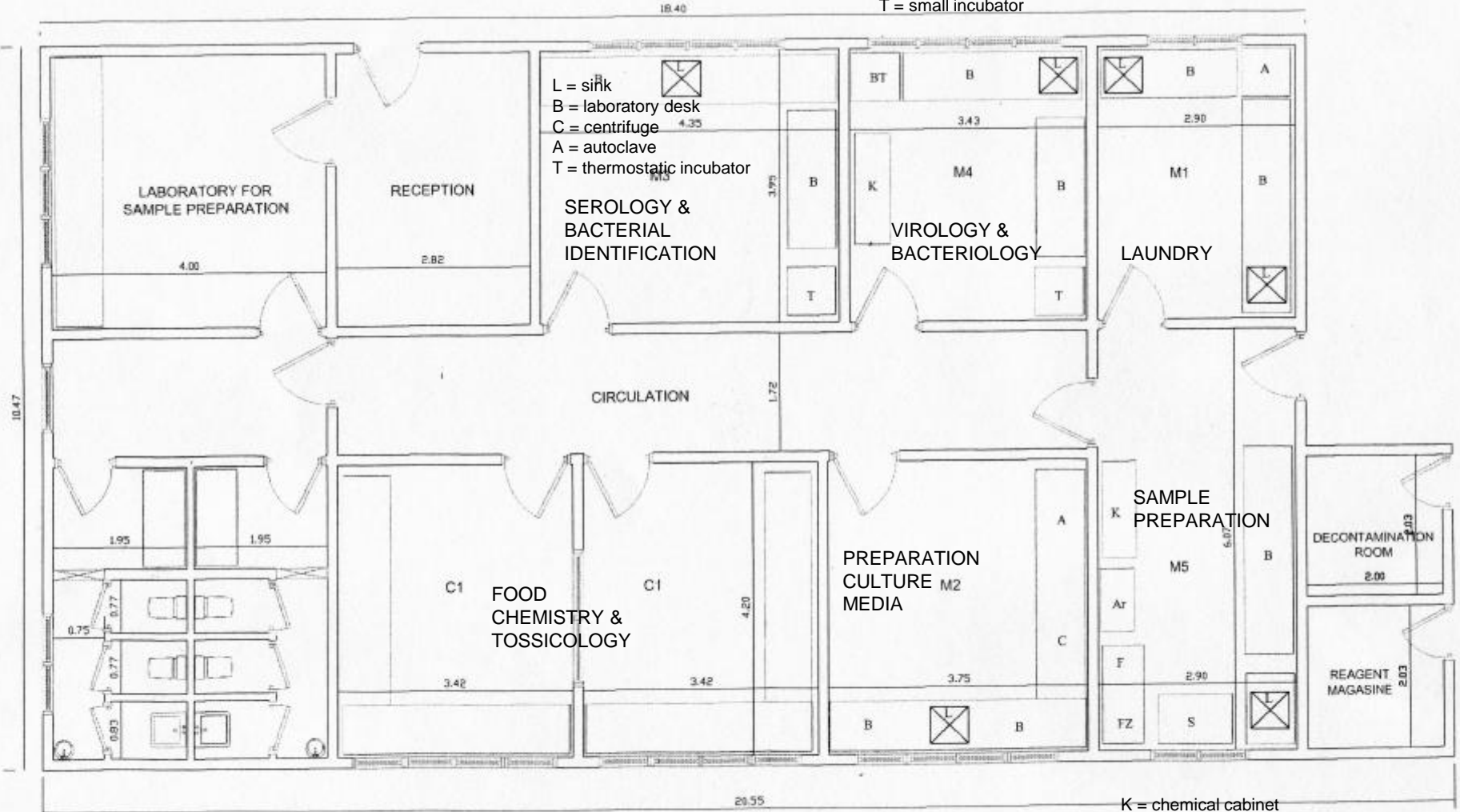
PLAN DE RENOVATION PROPOSE POUR LE BATIMENT 1 ANCIEN ENSA
